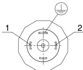
Рисунок В.3 — Нумерация контактов разъема GSP
