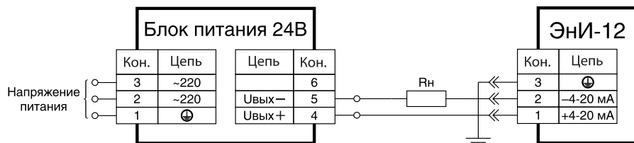
Рисунок В.1 — Подключение датчика
