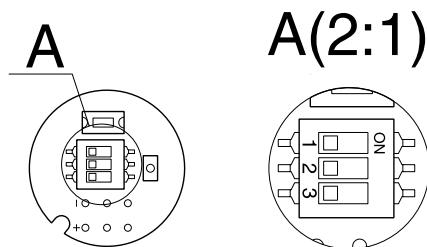
Рисунок 2.4 — Положение кнопок механического переключателя
