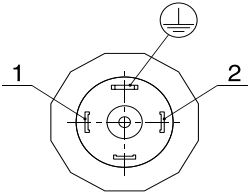
Рисунок В.3 — Нумерация контактов разъема GSP
