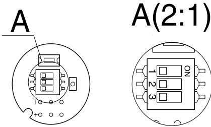
Рисунок 2.4 — Положение кнопок механического переключателя
