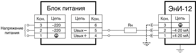
Рисунок В.1 — Подключение датчика
