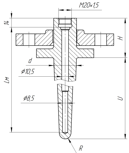
Рисунок А.48 – ГТ-704 исполнение Vanstone для ДТ с подвижным штуцером со ступенчатым внутренним диаметром
