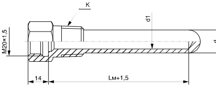
Рисунок А.10 — ГТ-702 цилиндрическая с конической резьбой для ДТ с подвижным штуцером
