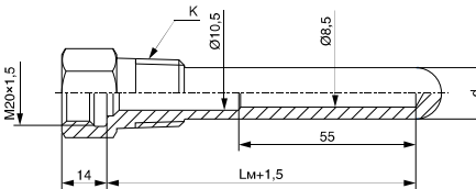
Рисунок А.12 — ГТ-702 цилиндрическая с конической резьбой для ДТ с подвижным штуцером со ступенчатым внутренним диаметром
