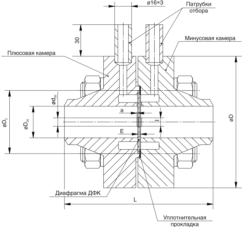
Рисунок Б.4 — Диафрагма ДФК
