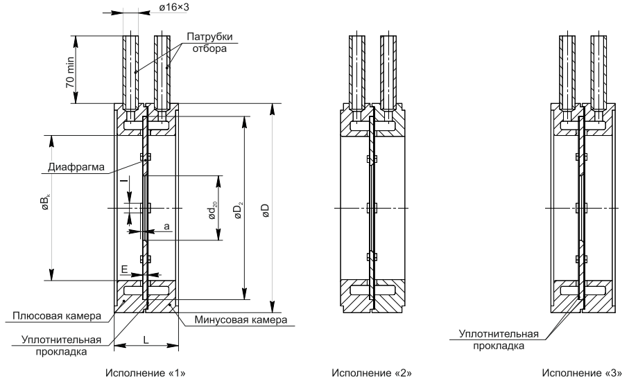
Рисунок Б.1 — Конструктивные исполнения камер ДКС
